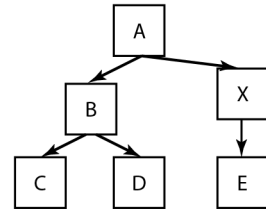
(c) Po całkowitym zainicjowaniu węzła X podłączamy X do A. Czytelnicy, którzy aktualnie są w węzle E, muszą odczytać starą wersję, natomiast czytelnicy w węzle A pobiorą nową wersję drzewa
