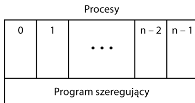
Rysunek 2.3. Najniższa warstwa systemu operacyjnego o strukturze procesów zarządzająca przerwaniem i szeregowaniem. Powyżej tej warstwy znajdują się sekwencyjne procesy
