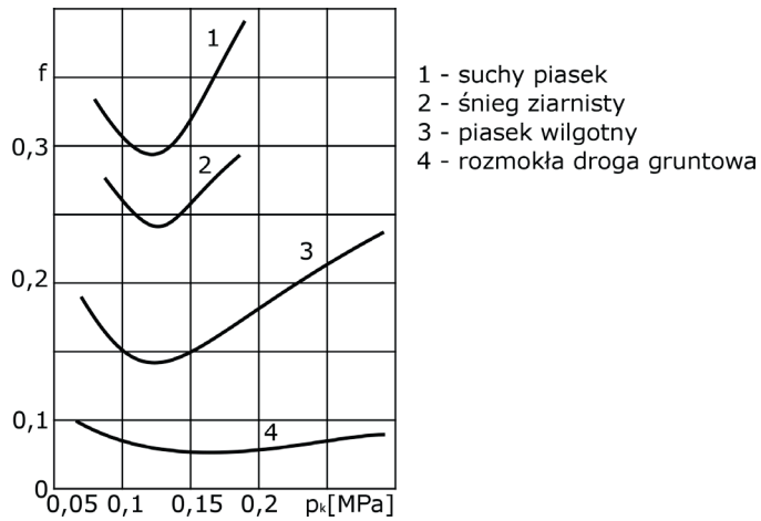
Rys. 4. Zależność współczynnika oporu toczenia f od ciśnienia powietrza w kole [23]
