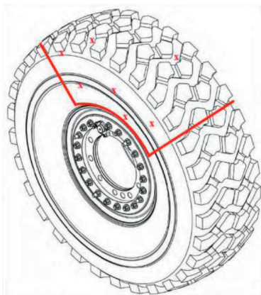
Rys. 8. Lokalizacja miejsc oddania strzału podczas badań wkładek nośnych run-flat (5 strzałów – bok opony, 2 strzały – bieżnik) [38]
