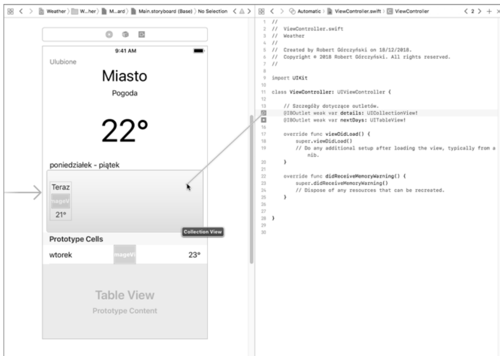
Rysunek 7.20. Połączenie outletu z elementem interfejsu użytkownika
