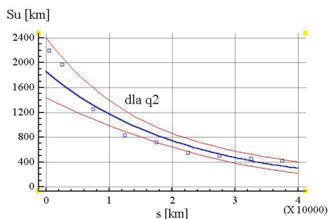
Rys. 13. Zależność S_u = f(s, q) , dla q_2 = 900-2600 [km/rok]
