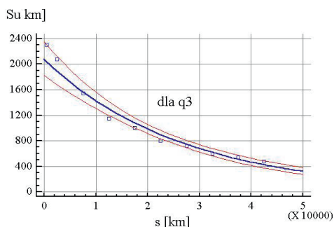
Rys. 14. Zależność S_u = f(s, q) , dla q_3 = 2600-4500 [km/rok]
