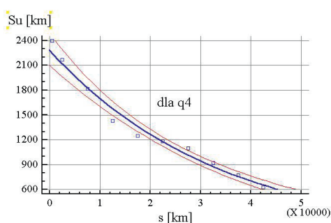
Rys. 15. Zależność S_u = f(s, q) , dla q_4 > 4500 [km/rok]
