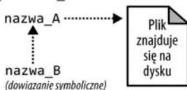
Rysunek 5. Dowiązania sztywne i symboliczne
