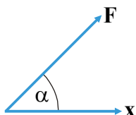
Rys. 014. Praca ( W ) jest iloczynem skalarnym siły ( \mathbf{F} ) i przemieszczenia ( \mathbf{x} ).
