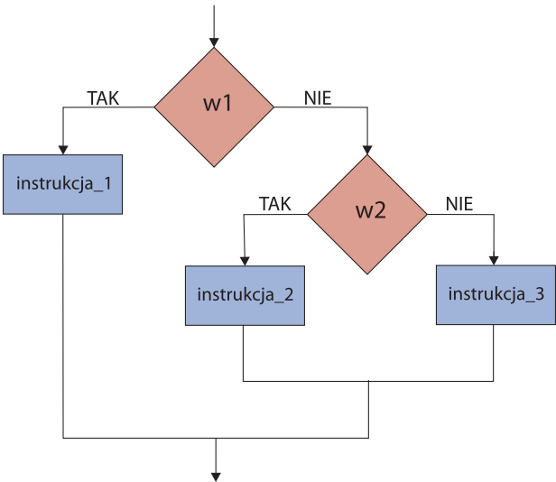
Rysunek 7.4. Schemat blokowy złożonej instrukcji warunkowej
