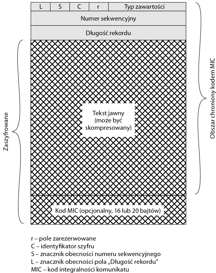
Rysunek 4.17. Format rekordu WTLS
