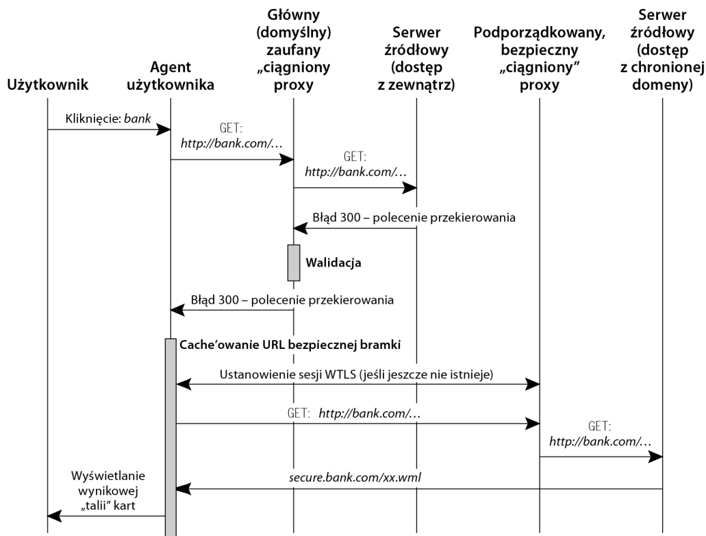
Rysunek 4.22. Przykład całościowego zabezpieczenia transmisji WAP na poziomie warstwy transportowej, z wykorzystaniem przekierowania HTTP
