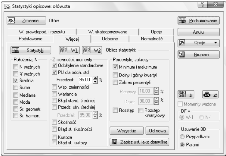
Rysunek 4.8. Okno wyboru statystyk opisowych
