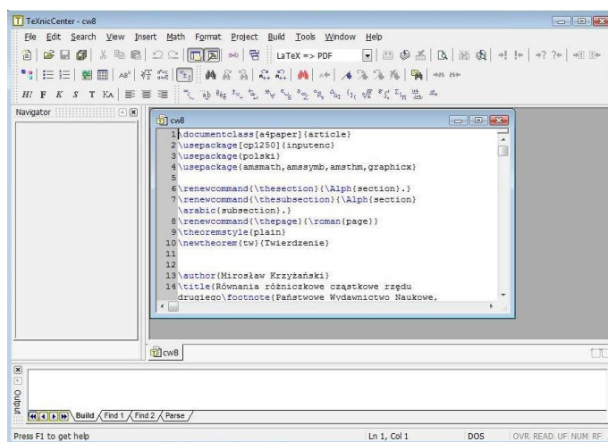
TeXnicCenter
