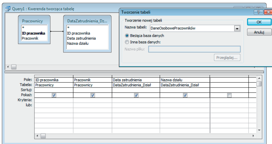
Rysunek 3.15. Projekt kwerendy tworzącej tabelę
