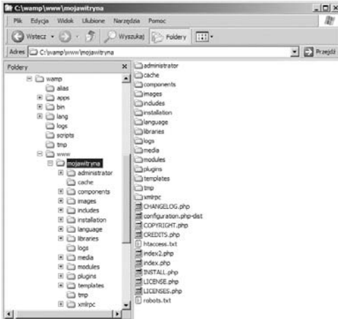
Rysunek 1.1. Struktura katalogu głównego systemu Joomla
