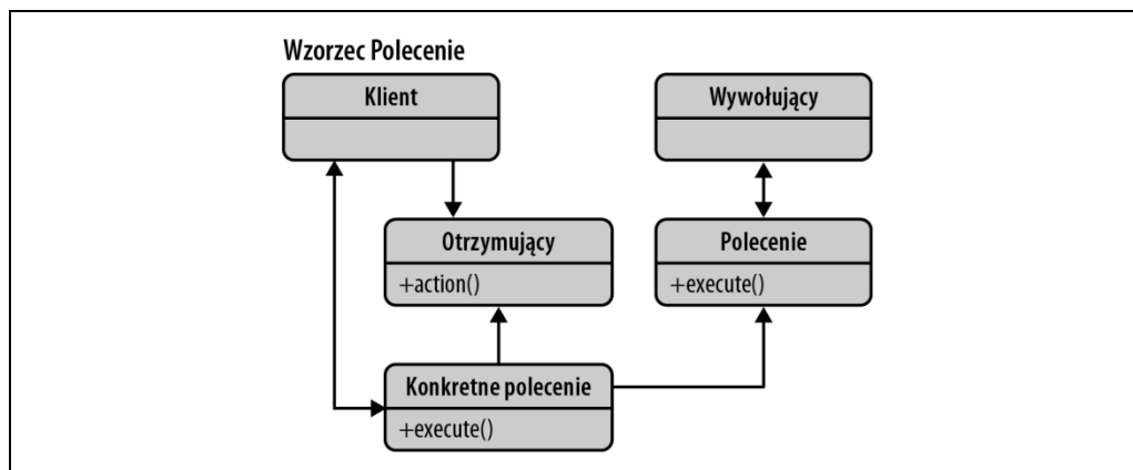
Rysunek 7.12. Wzorec Polecenie
