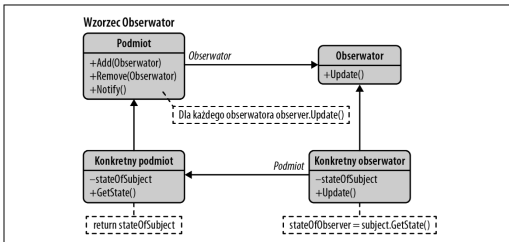
Rysunek 7.9. Wzorzec Obserwator
