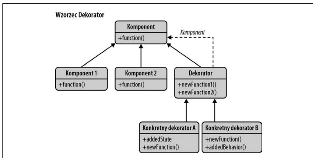
Rysunek 7.7. Wzorec Dekorator
