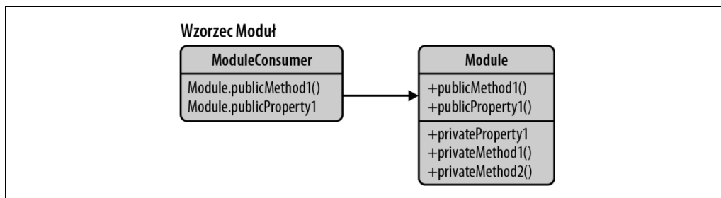
Rysunek 7.2. Wzorzec Moduł
