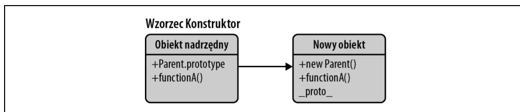
Rysunek 7.1. Wzorec Konstruktor
