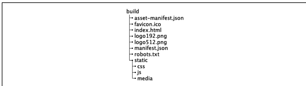
Rysunek 1.2. Wygenerowane treści umieszczone w katalogu build
