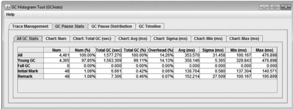
Rysunek 4.1. Statystyki przestojów mechanizmów odzyskiwania pamięci w GCHisto
