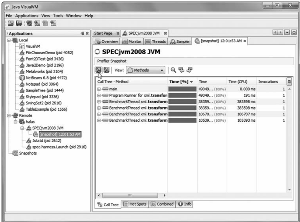
Rysunek 4.13. Zapisywanie zrzutu ekranu
