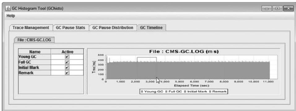
Rysunek 4.4. Powiększanie obszaru wykresu w zakładce GC Timeline
