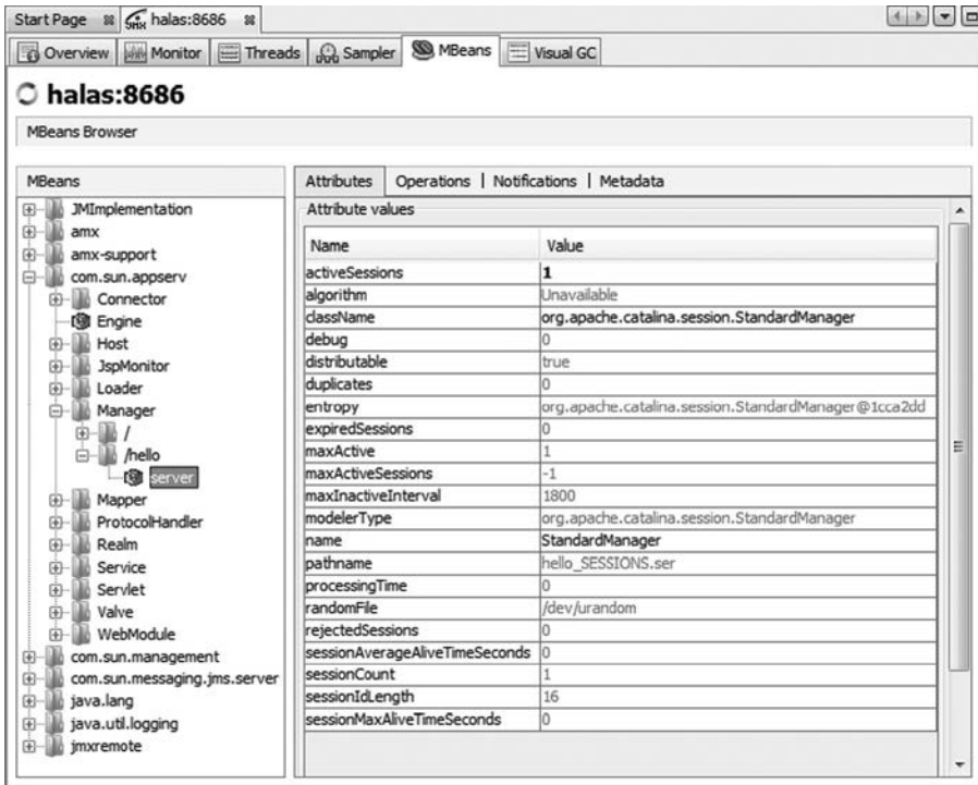
Rysunek 4.20. MBeany GlassFish
