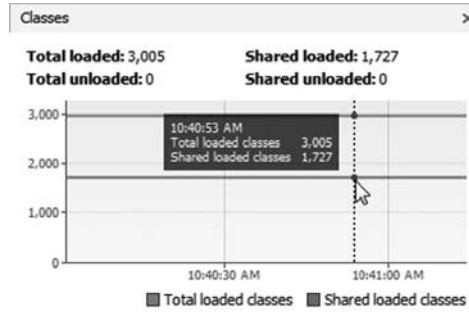
Rysunek 4.18. Zaobserwowane współdzielenie klas
