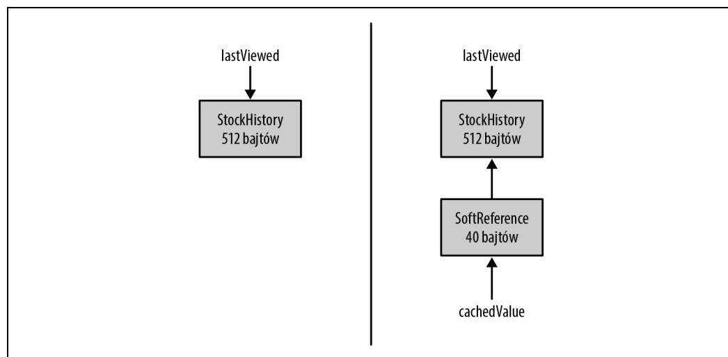
Rysunek 7.6. Pamięć zajmowana przez niezdefiniowane odwołanie
