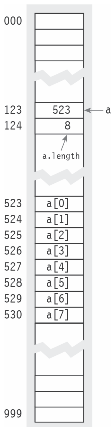
Rysunek 1.25. Reprezentacja w pamięci
