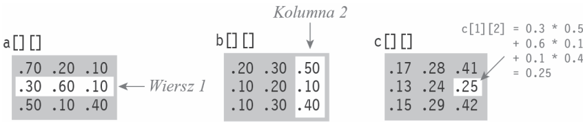
Rysunek 1.35. Mnożenie macierzy
