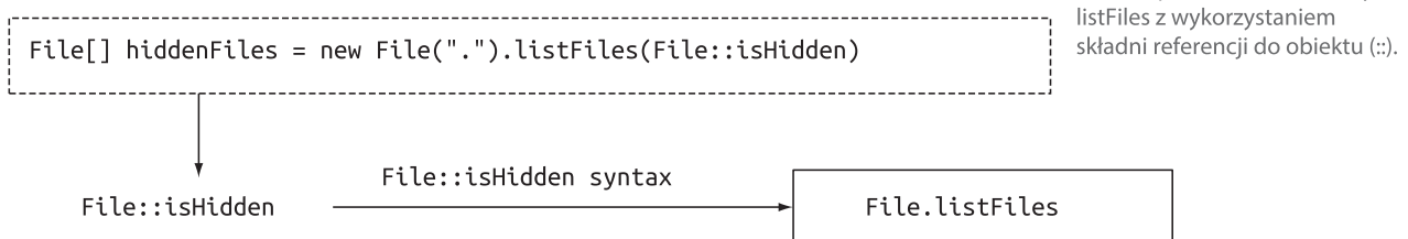
Rysunek 1.4 Przekazywanie do metody listFiles referencji do metody File::isHidden
