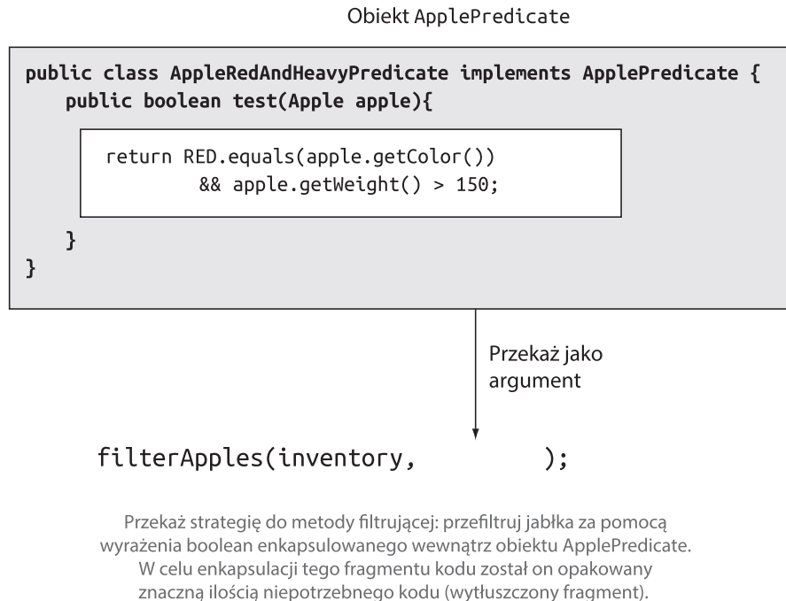
Rysunek 2.2 Parametryzowanie zachowania metody filterApples i przekazywanie różnych strategii filtrowania
