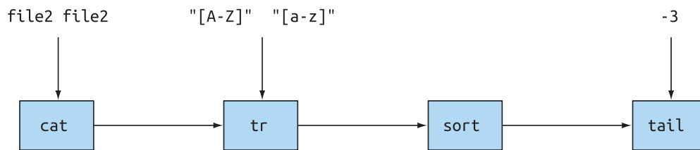
Rysunek 1.2 Polecenia systemu Unix operujące na strumieniu
