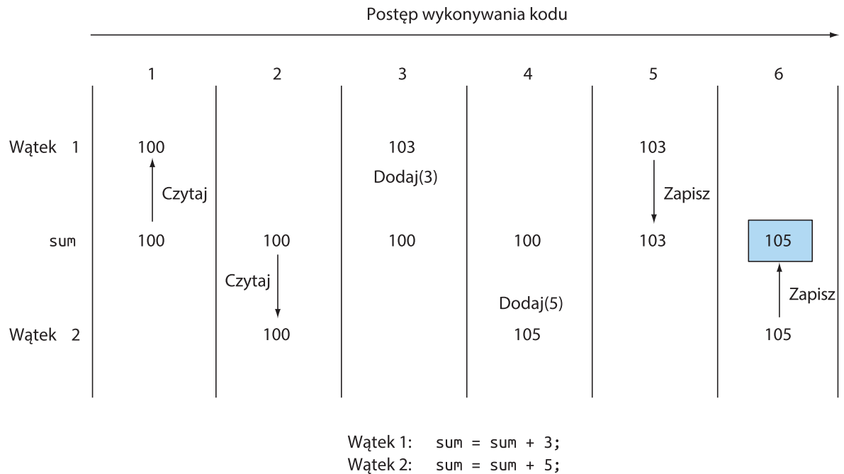
Rysunek 1.5 Możliwy problem z dwoma wątkami próbującymi dodać liczbę do współdzielonej zmiennej sum . Wynikiem jest 105 zamiast oczekiwanego 108.
