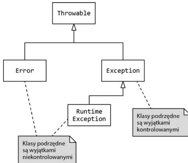
Rysunek 5.1. Hierarchia wyjątków
