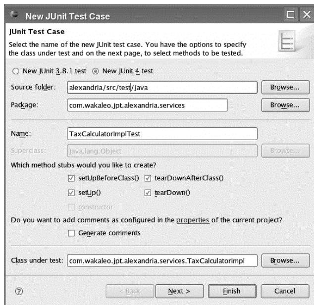
Rysunek 10.3. Tworzenie w środowisku Eclipse nowego testu frameworku JUnit 4
