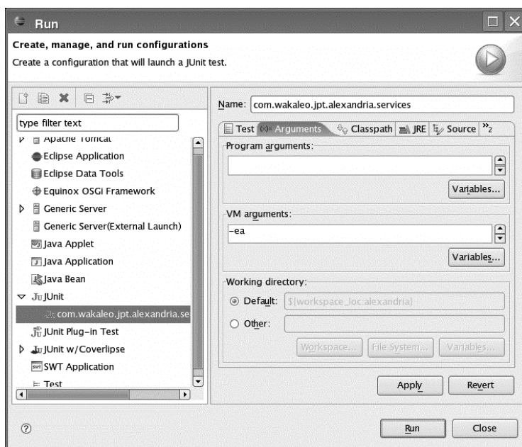
Rysunek 10.1. Konfigurowanie testów frameworku JUnit 4, aby korzystały z operacji asercji
