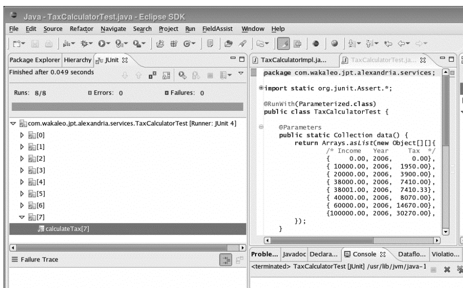
Rysunek 10.2. Uruchamianie testów frameworku JUnit 4 z poziomu środowiska Eclipse
