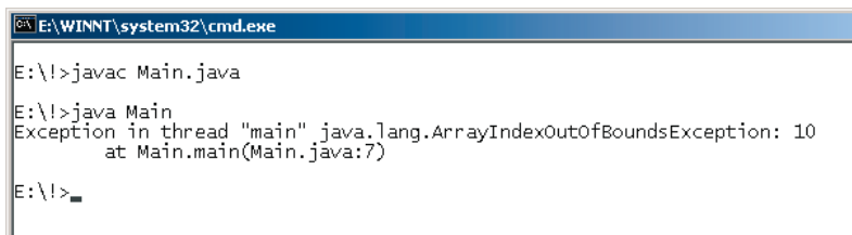
Rysunek 2.3. Próba odwołania się do nieistniejącego elementu tablicy
