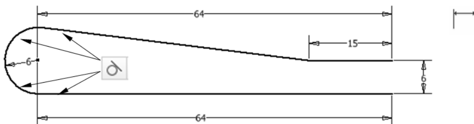
Rysunek 4.59. Wymiarowanie szkicu i dodawanie wiązania styczności
