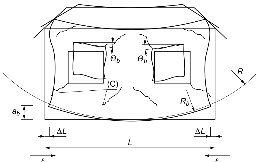
Rys. 1.8. Schemat deformacji i uszkodzeń ścian na wklęsłej części niecki [12]
