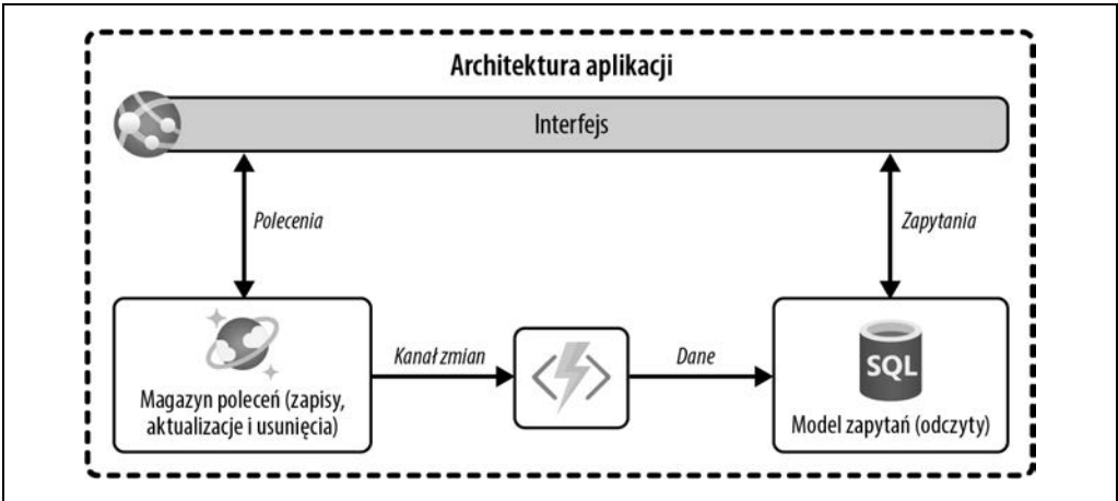
Rysunek 4.2. Aplikacja korzystająca z wzorca CQRS oddziela zapytania i polecenia za pomocą dwóch różnych modeli danych: modelu poleceń przeznaczonego do transakcji oraz modelu zapytań przewidzianego do odczytów
