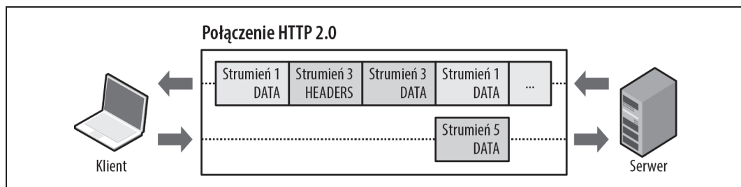
Rysunek 12.9. Multipleksacja żądań i odpowiedzi we współdzielonym połączeniu HTTP 2.0
