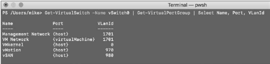
RYSUNEK 5.17. Korzystanie z CLI pomaga sprawdzić, czy grupa portów i port VMkernel to oddzielne obiekty
