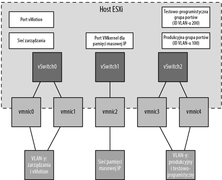
RYSUNEK 5.42. Użycie fizycznie oddzielnej sieci dla pamięci masowej IP ogranicza redukcję liczby przełączników virtualnych i uplinków
