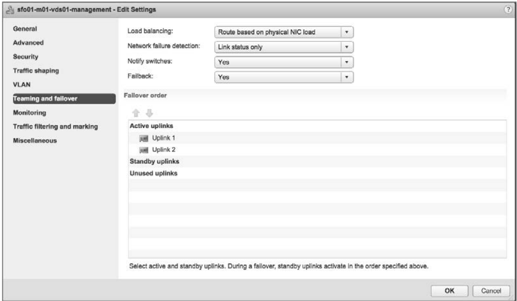
RYSUNEK 5.56. Ustawienia Teaming and failover w oknie dialogowym Edit Settings dla rozproszonej grupy portów zapewniają opcje dla modyfikowania sposobu używania uplinków przez tę rozproszoną grupę portów
