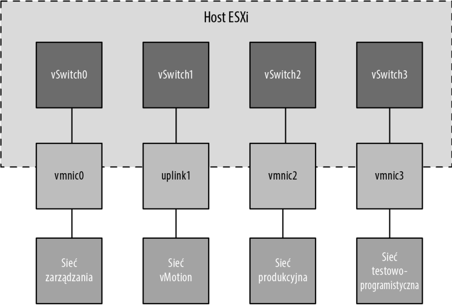
RYSUNEK 5.24. Obsługa wielu sieci bez VLAN-ów może zwiększyć liczbę wymaganych przełączników wirtualnych i uplinków oraz ilość okablowania
