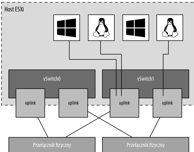
RYСУNEK 5.32. Reguła równoważenia obciążenia oparta na wirtualnych portach pochodzenia przypisuje każdy port przełącznika wirtualnego do określonego uplinku. Przełączenie awaryjne na inny uplink ma miejsce wtedy, gdy jedna z fizycznych kart sieciowych doznaje awarii
