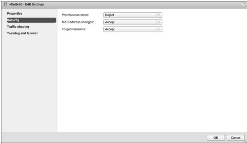
RYСУNEK 5.74. Domyślny profil bezpieczeństwa dla przełącznika standardowego nie dopuszcza trybu mieszanego, zezwala na zmiany adresów MAC i sfałszowane transmisje
