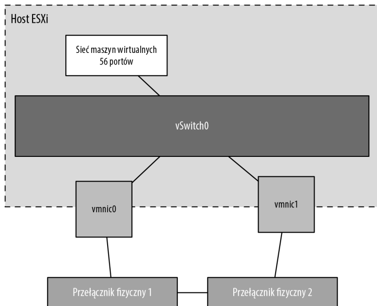
RYСУNEK 5.22. Przełącznik wirtualny z grupą portów maszyn wirtualnych wykorzystuje powiązane z nim fizyczne karty sieciowe do ustanowienia bezpośrednich połączeń z przełącznikami fizycznymi
