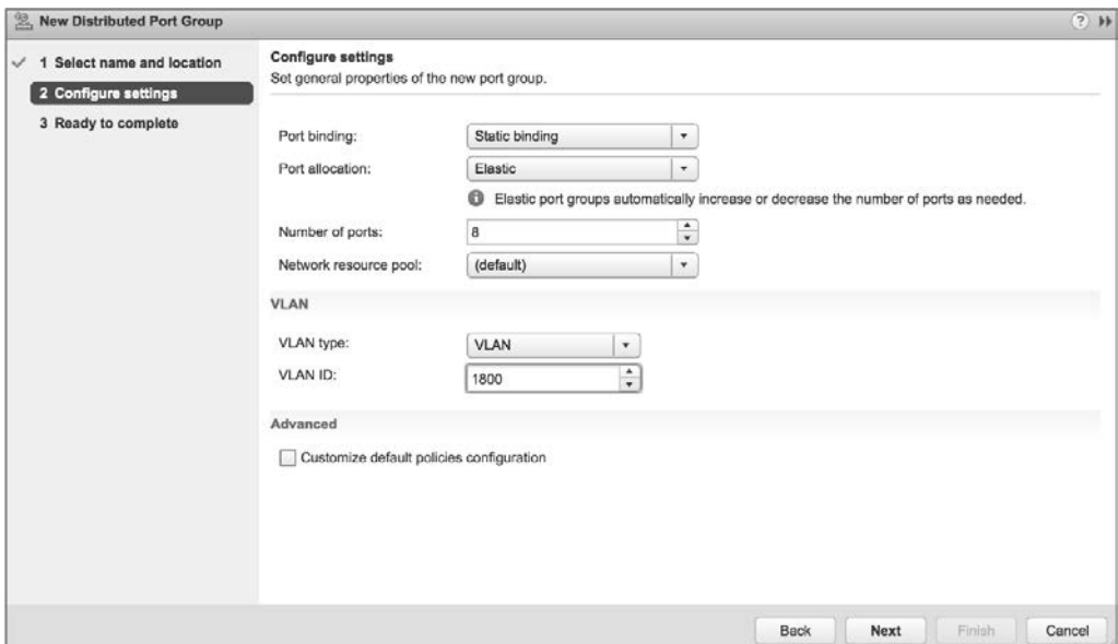
RYSUNEK 5.51. Kreator nowej rozproszonej grupy portów oferuje szerokie możliwości dostosowywania ustawień tej grupy
