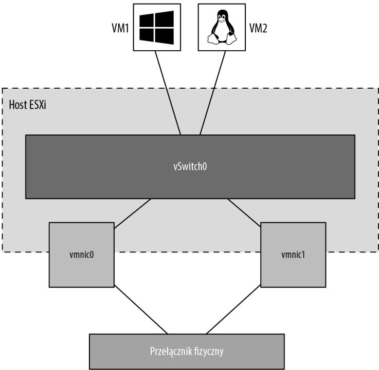
RYSUNEK 5.7. Przełącznik wirtualny korzystający z grupy kart sieciowych ma dostępnych wiele interfejsów do transferu danych. Grupowanie kart sieciowych oferuje redundancję i dystrybucję obciążenia
