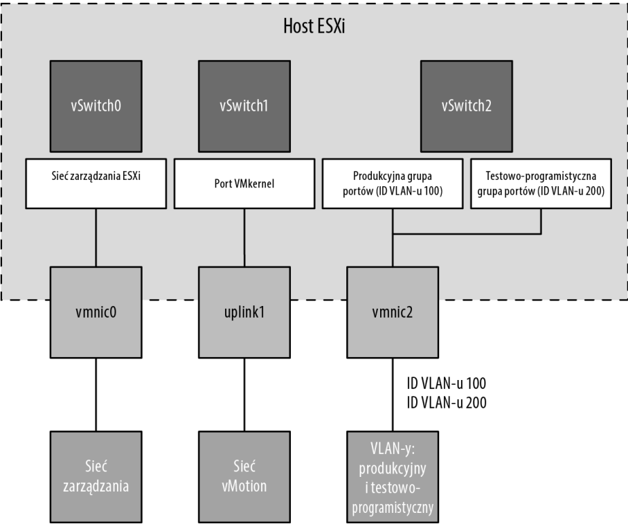
RYSUNEK 5.25. VLAN-y mogą zmniejszyć liczbę wymaganych przełączników wirtualnych i uplinków oraz ilość okablowania
