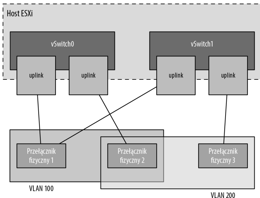
RYСУNEK 5.30. Wszystkie fizyczne karty sieciowe w grupie muszą przenosić te same VLAN-y
