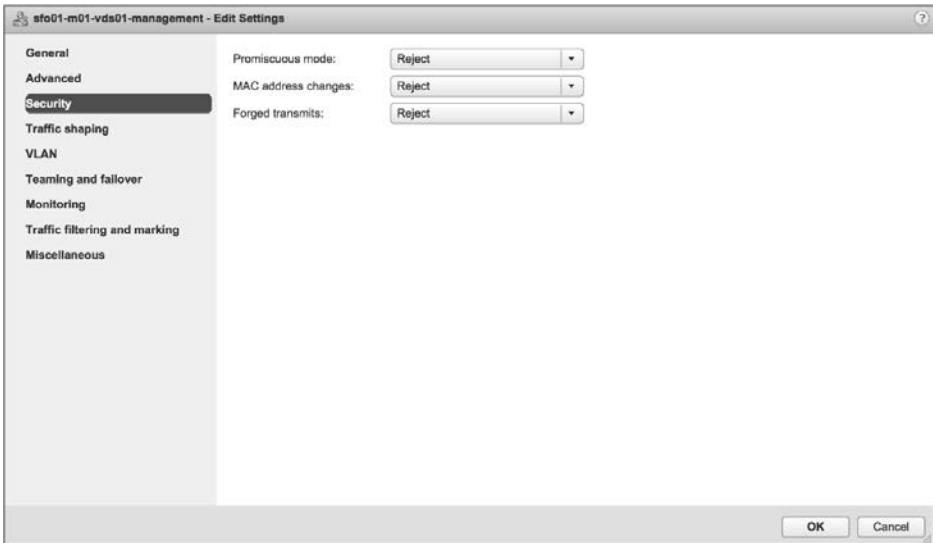
RYСУNEK 5.75. Domyślny profil bezpieczeństwa dla rozproszonej grupy portów na przełączniku rozproszonym nie dopuszcza również zmian adresów MAC i sfałszowanych transmisji
