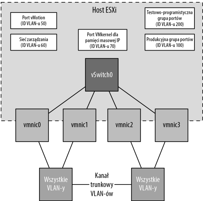
RYSUNEK 5.43. Dzięki użyciu grup portów i VLAN-ów na przełącznikach wirtualnych wymagana byłaby jeszcze mniejsza liczba przełączników wirtualnych i uplinków
