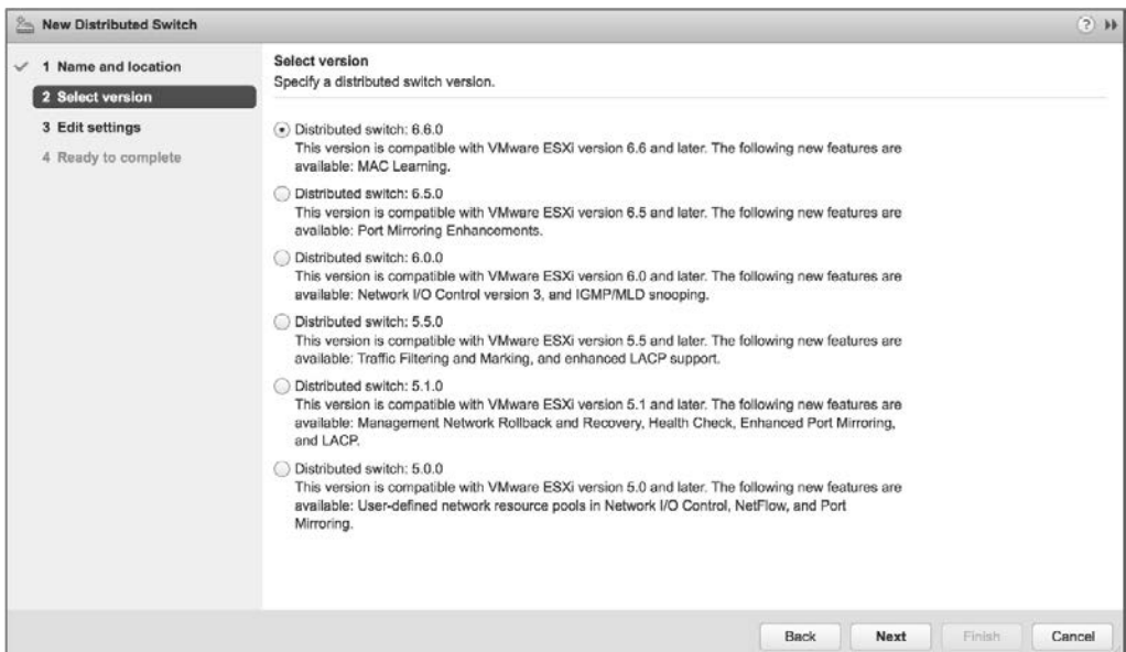
RYСУNEK 5.44. Jeśli chcesz zapewnić wsparcie dla wszystkich funkcjonalności dostępnych w vSphere 6.7, musisz użyć wersji 6.6.0 przełącznika rozproszonego
