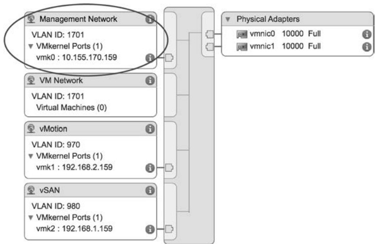
RYСУNEK 5.4. Możesz tworzyć przełączniki wirtualne posiadające jednocześnie oba typy połączeń
