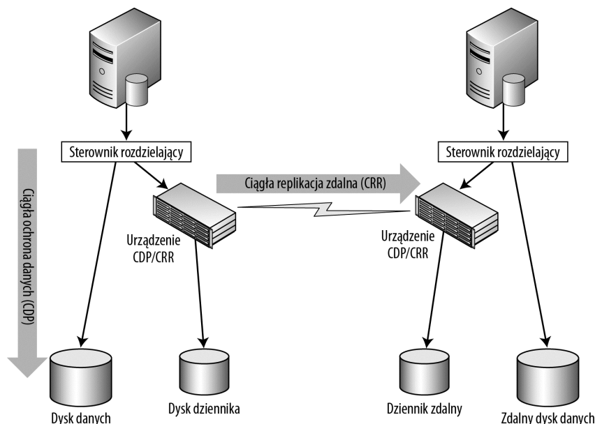
Rysunek 5.14. Technologia CDP i CRR
