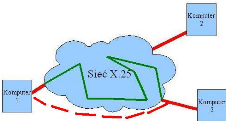
Rysunek 5.3 – Połączenie logiczne i fizyczne w sieci X.25
