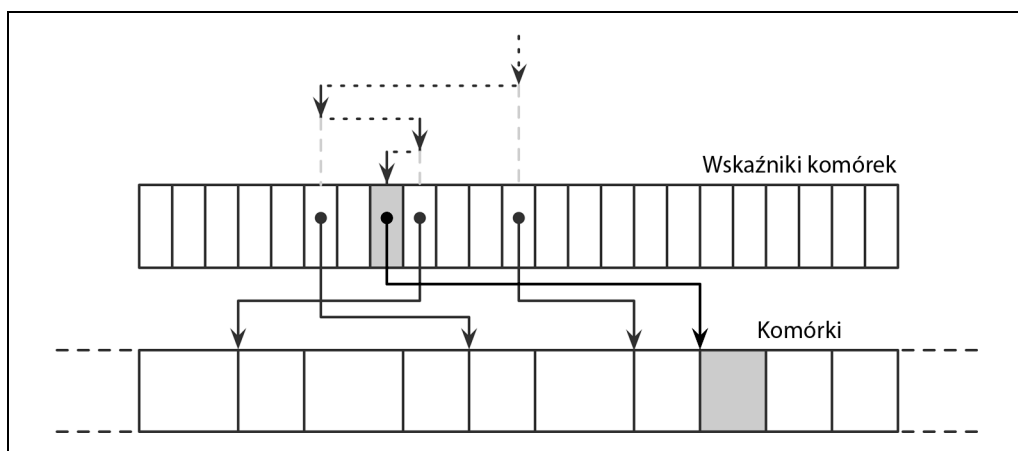
Rysunek 4.7. Wyszukiwanie binarne ze wskaźnikami pośrednimi. Szukany element jest zaznaczony szarym kolorem. Kropkowane strzałki reprezentują wyszukiwanie binarne poprzez wskaźniki komórek. Linie ciągłe reprezentują dostępy do danych, które idą za wskaźnikami komórek i są niezbędne do porównania wartości komórki z wyszukiwanym kluczem
