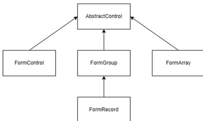
RYSUNEK 1.3. Struktura bazowych klas formularzy
