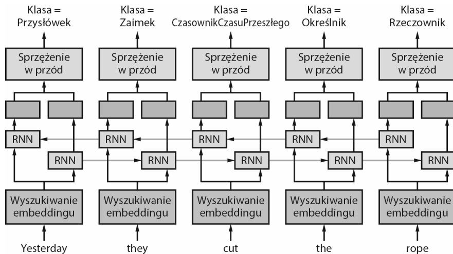
RYСУNEK 24.4. Dwukierunkowa sieć RNN dla tagowania części mowy
