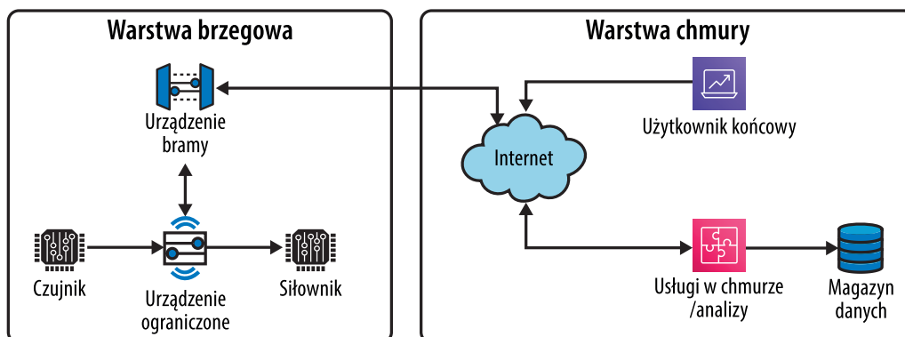
Rysunek P-1 Koncepcyjny projekt architektury systemu IoT
