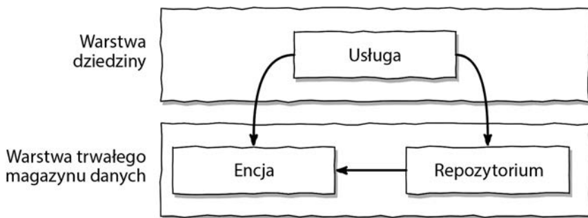
Rysunek 2.2. Przykład użycia encji bazy danych w warstwie dziedziny prowadzi do silnego jej powiązania z warstwą trwałego magazynu danych
