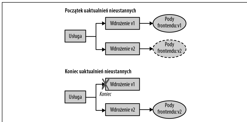
Rysunek 5.1. Uaktualnienia nieustanne w Kubernetes
