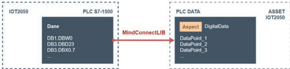
RYSUNEK 7.7. Mapowanie fizycznych urządzeń i zestawu danych na logiczne assety i aspekty w środowisku MindSphere
