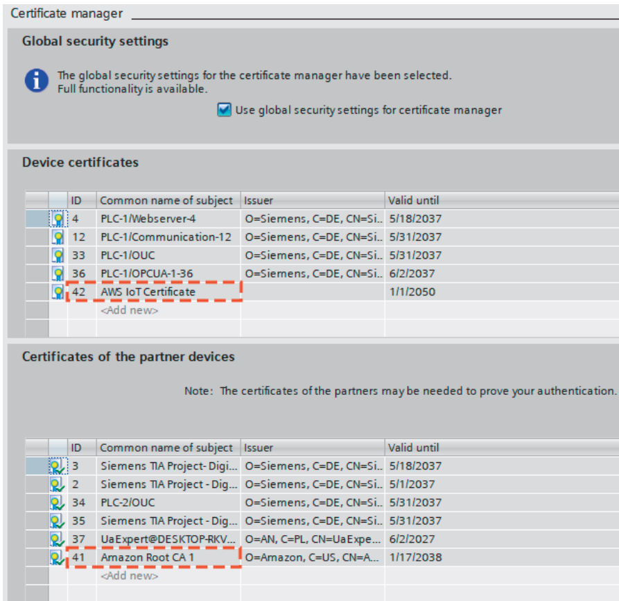
RYСУNEK 7.30. Przypisanie certyfikatów urządzenia i chmury AWS do lokalnego menedżera w urządzeniu
