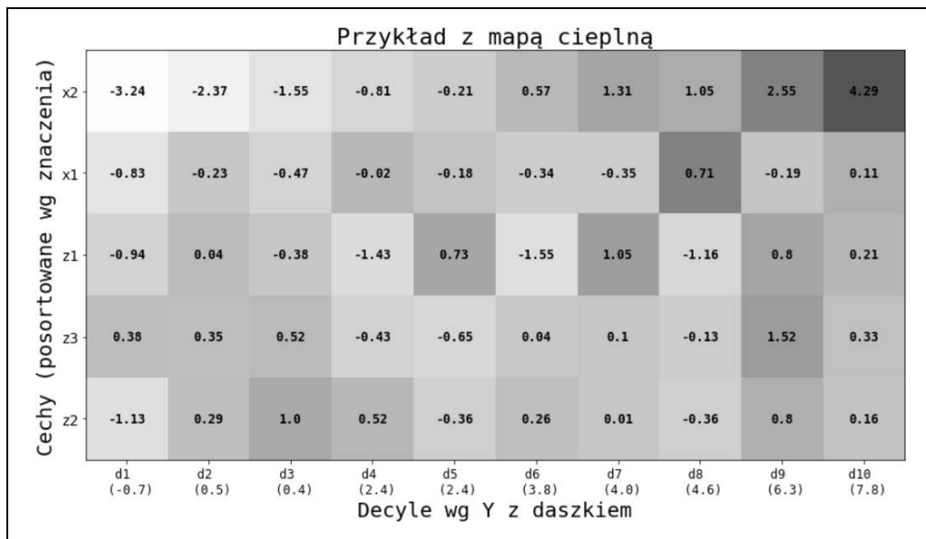
Rysunek 13.8. Mapa cieplna cech dla wcześniejszego przykładu z symulacją
