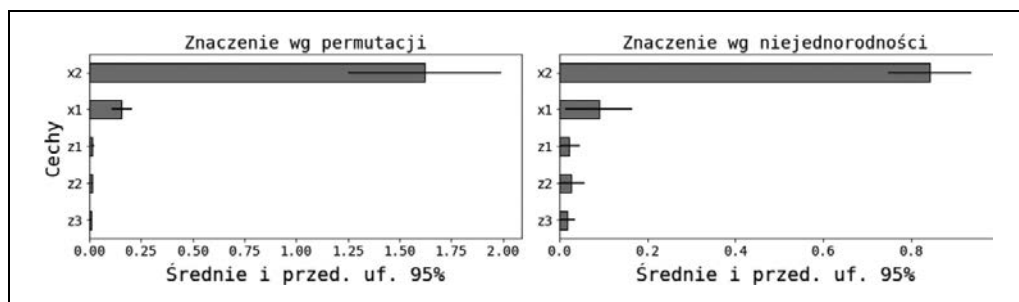
Rysunek 13.7. Znaczenie cech w symulowanym modelu opartym na regresji ze wzmacnianiem gradientowym
