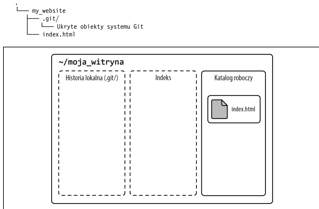
Rysunek 1.2. Początkowe repozytorium
