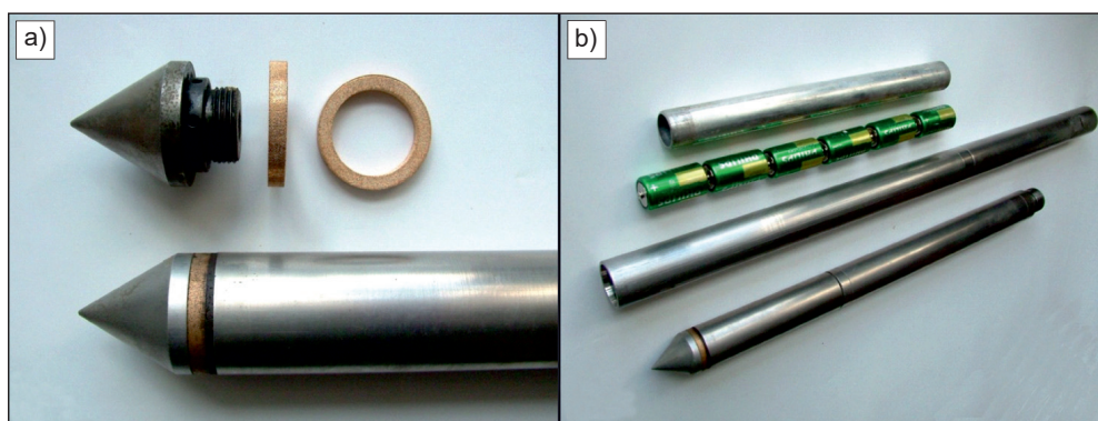
Ryc. 4.2. Końcówka badawcza; a) stożek, filtr porowy końcówki CPTu, b) końcówka CPTu wraz z modułem zasilania bateriami
