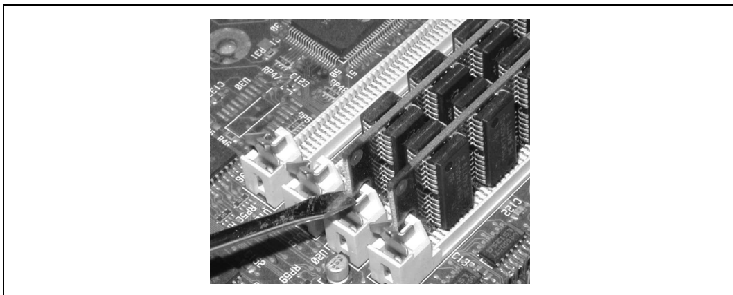
Rysunek 5.5. Zastosowanie małego śrubokręta do podważenia zatrzasków przy jednoczesnym łagodnym nacisku na moduł
