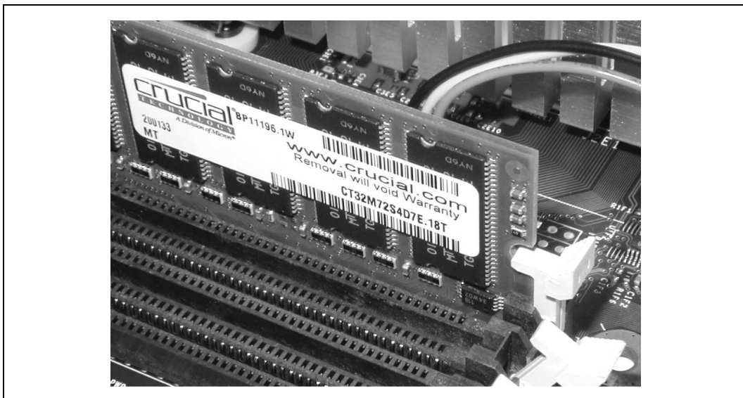
Rysunek 5.7. Dzwignie prowadnic ustawiają się pionowo, gdy moduł pamięci znajduje się we właściwym położeniu
