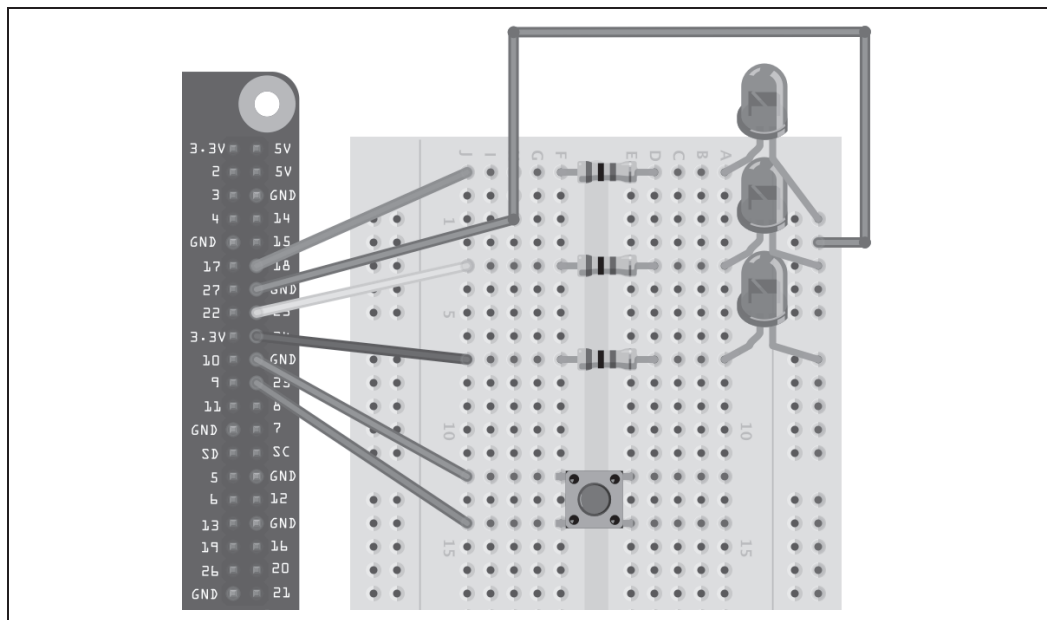
Rysunek 16.1. Schemat obwodu sterowanego za pośrednictwem strony Web
