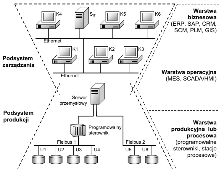
Rysunek 2.2. Model infrastruktury systemów informatycznych składających się na rozproszony system sterowania; K1 do K6 — klienci komputerowej sieci Ethernet; SIT — serwer systemów informatycznych; U1 do U6 — urządzenia automatyki przemysłowej
