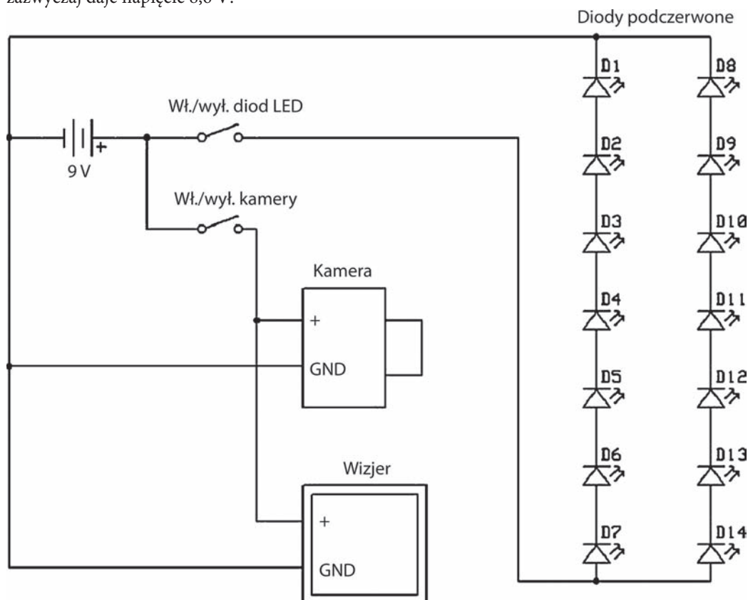
RYСУNEK 10.36. Połączenie wszystkich komponentów ze źródłem zasilania
