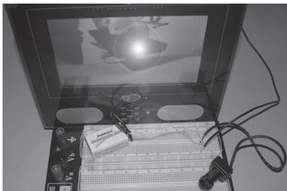
RYСУNEK 10.9. Testowanie reakcji kamery na promieniowanie podczerwone
