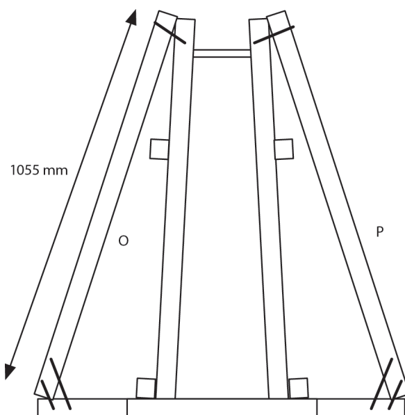
RYSUNEK 2.8. Podstawa i rozpórki boczne
