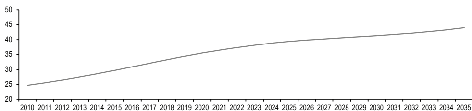
Wykres 1. Prognoza wskaźnika obciążenia demograficznego dla Polski
