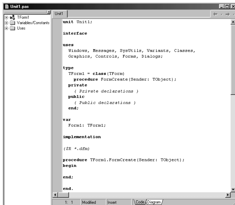
Rysunek 4.1. Okno edycji kodu głównego modułu aplikacji
