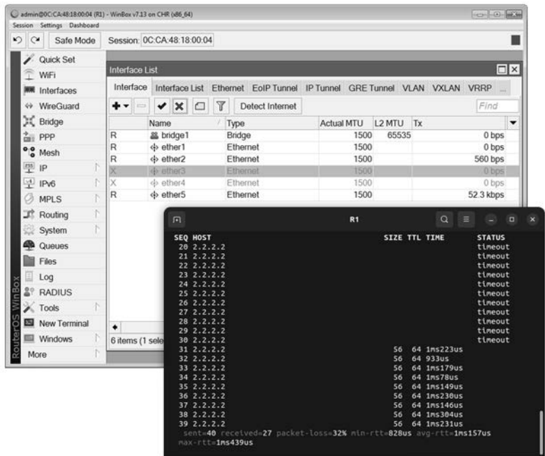
RYSUNEK 1.13. Router R1, test działania funkcji testu bramy
