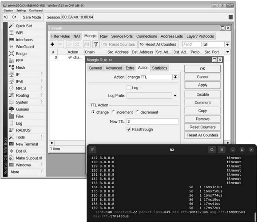
RYSUNEK 1.22. Router R2, odzyskanie połączenia z siecią Internet
