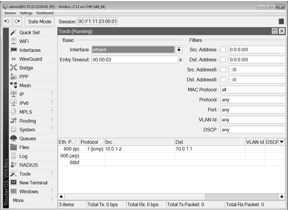
RYSUNEK 1.35. Router R1, interfejs ether4, rejestrowanie ruchu sieciowego
