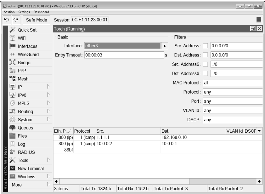
RYSUNEK 1.34. Router R1, interfejs ether3, rejestrowanie ruchu sieciowego
