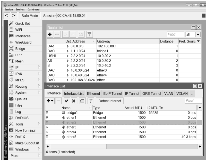
RYСУNEK 1.17. Router R1, wyłączenie interfejsu ether2
