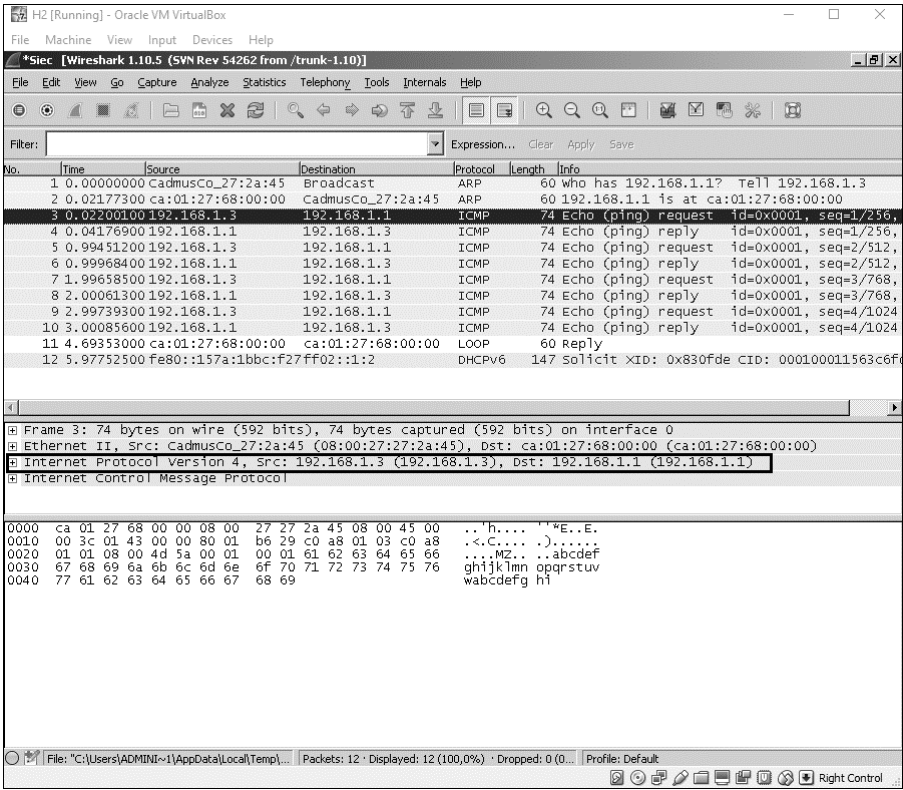
Rysunek 4.13. Przechwycona komunikacja ze stacji H2 do routera
