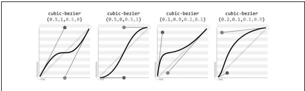
Rysunek 17.4. Cztery krzywe Béziera oraz wartości funkcji cubic-bezier() (na podstawie http://cubic-bezier.com )
