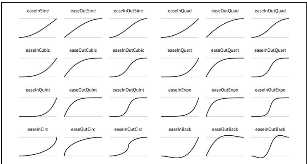
Rysunek 17.5. Przydatne funkcje Béziera opracowane przez innych autorów (ze strony http://easings.net )
