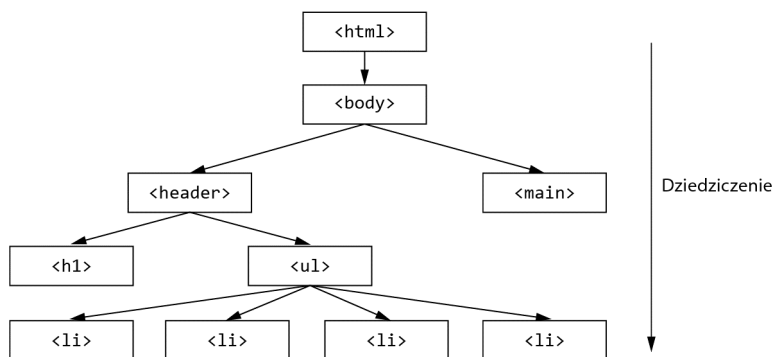
Rysunek 1.8. Dziedziczone właściwości są przekazywane w dół drzewa modelu DOM od węzłów nadrzędnych do ich węzłów podrzędnych
