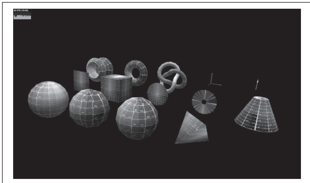
Rysunek 4.1. Przykłady obiektów geometrycznych biblioteki Three.js. Od lewej i od przodu: sfera, dwudziestościan, ośmiościan, czworoszczan; płaszczyzna, kostka, koło, pierścienie, cylinder; „tokarka”, torus i węzeł z torusa; osie x, y i z
